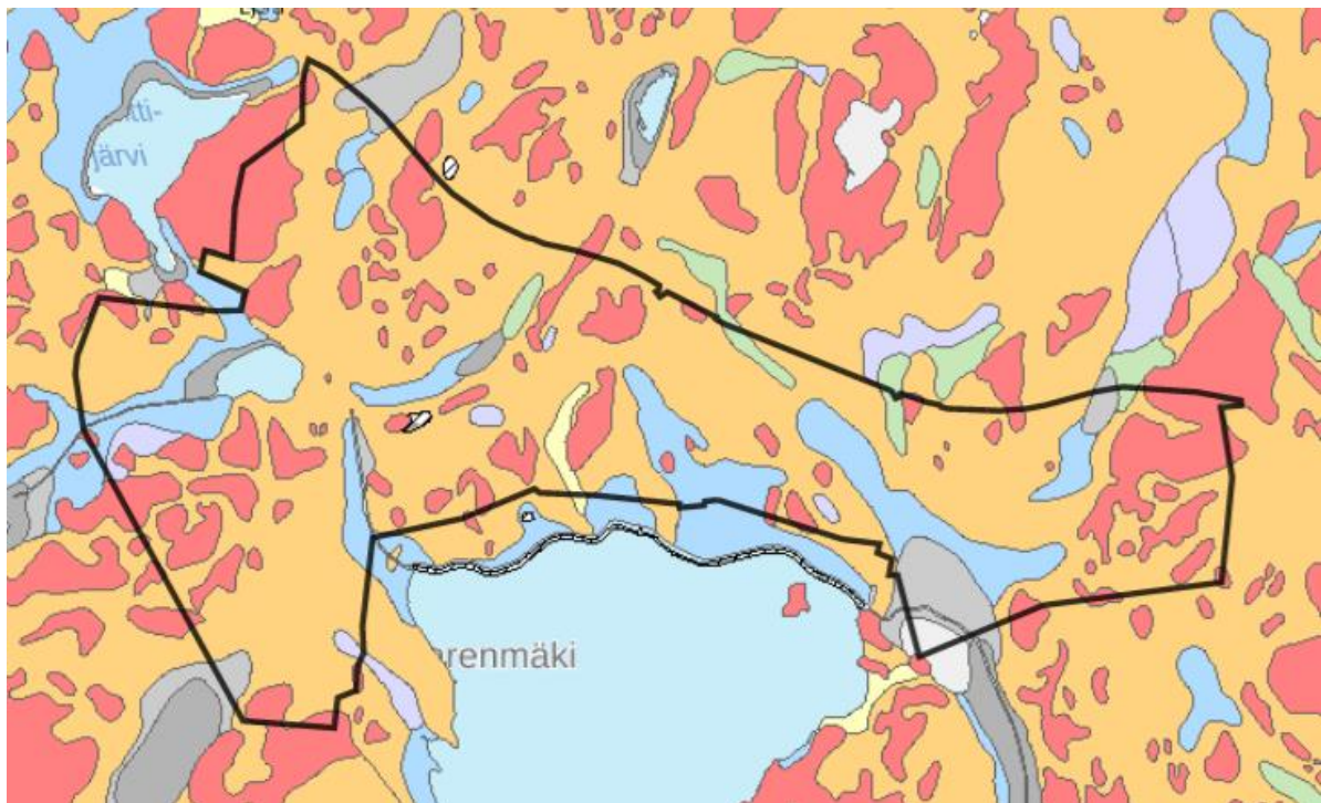
Kuva 8. Suunnittelualueen maaperä (1:20 000): punainen väri osoittaa kalliomaata, tummansininen väri savimaata, oranssi hienoainemoreenia, vihreä hiekkaa, vaaleansininen järveä. (GTK 2021)
