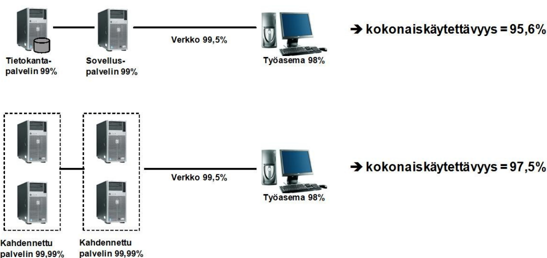
Kuva 7 Käytettävyyyslaskelma
